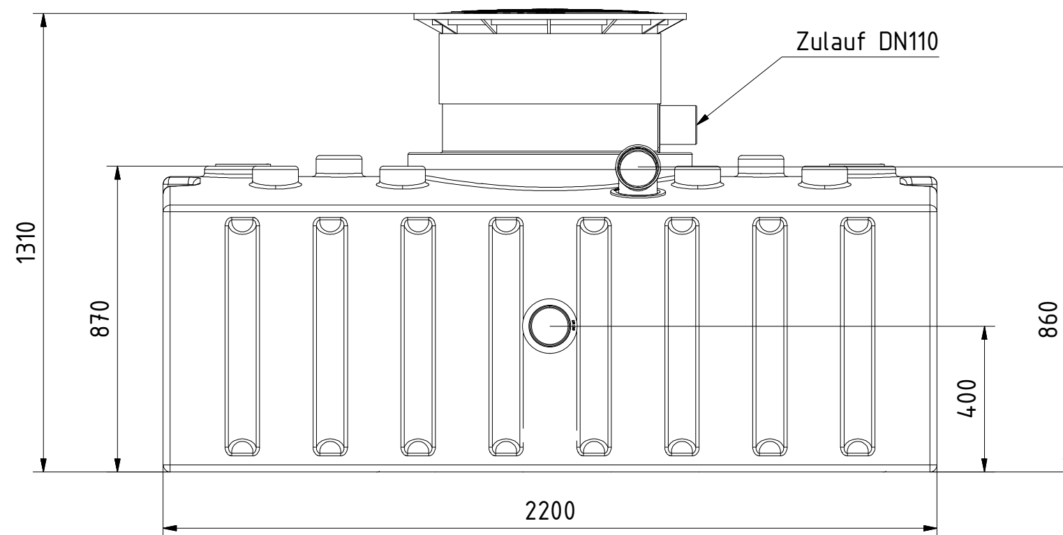
Seitenansicht
