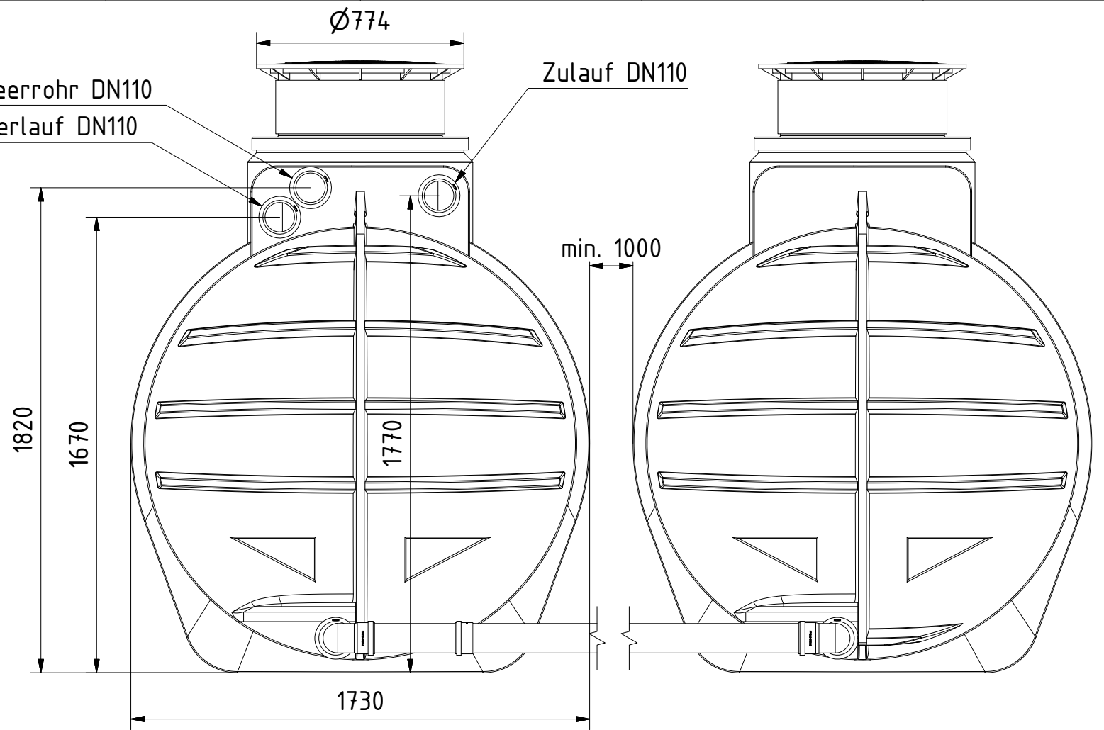
Frontansicht
