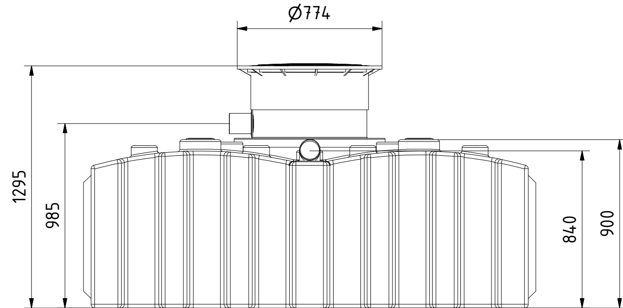
Frontansicht
