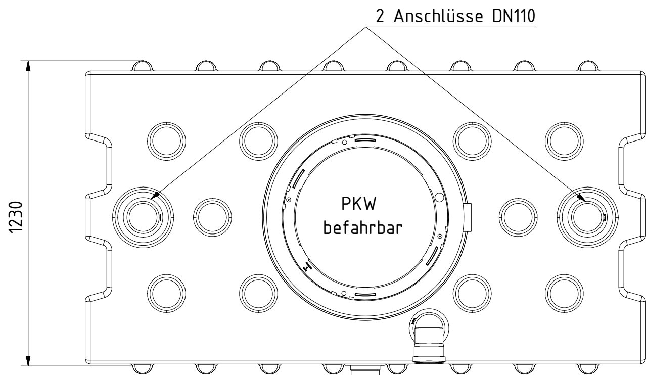
Draufsicht
