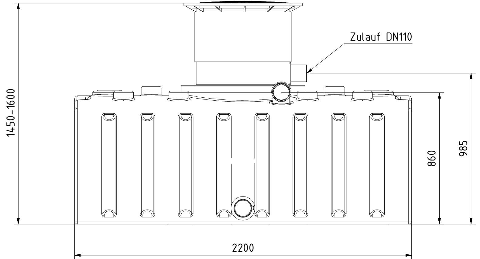
Seitenansicht
